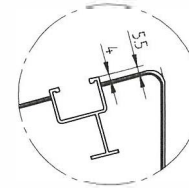
DETTAGLIO A
