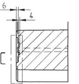
SEZIONE B-B
